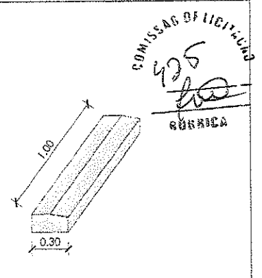
5 SECCÃO - MEIO FIO ESC.: 1/25 5 ISOMETRICO - MEIO FIO ESC.: 1/20
