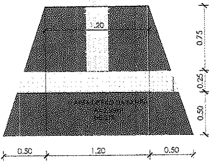
1 RAMPA - ACESSIVEL ESC.: 1/20
